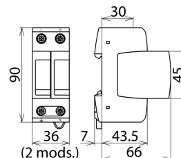
Dimensiones del DG M TT 2P 275
