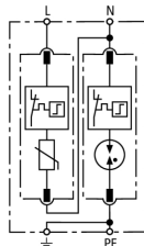
Esquema del DG M TT 2P 275
